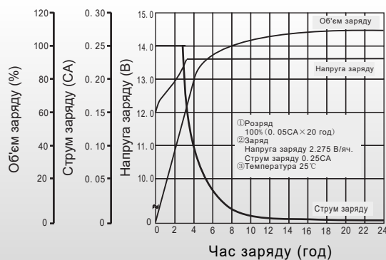
Характеристики заряду
