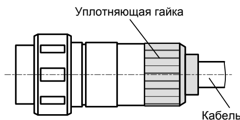
Рис.38. Кабельный разъем.
