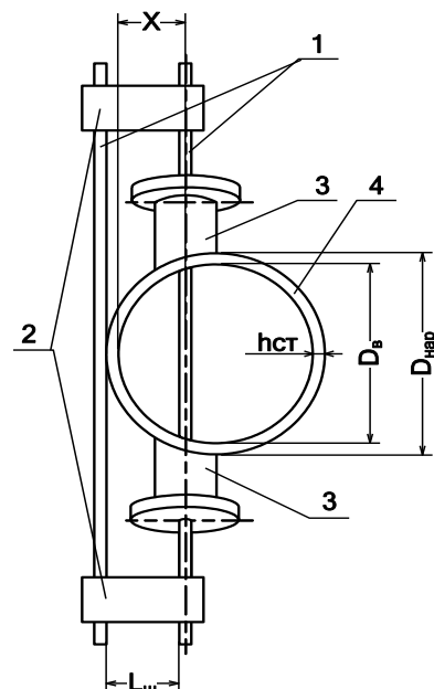
б) определение смещения оси акустического канала
