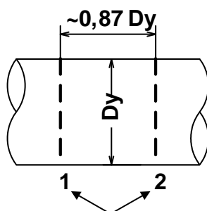
Рис.3. Положение сечений для размещения ПЭА на ИУ.
