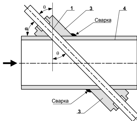
а) положение монтажных патрубков ПЭА на ИУ
