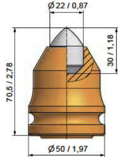
■ BKH85 B47K22-H/2
