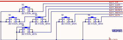
数码管电路
