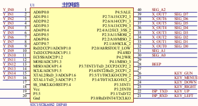
主控电路
