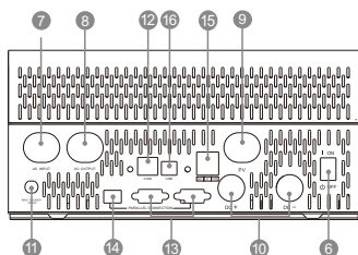
Паралельна модель 5,5 кВт
