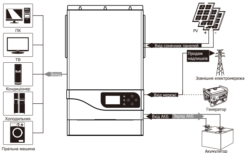
Рисунок 1 Гібридна система живлення
