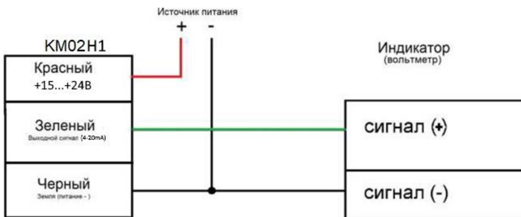
Рис1. Схема подключения KM02H1 к прибору(индикатору).
