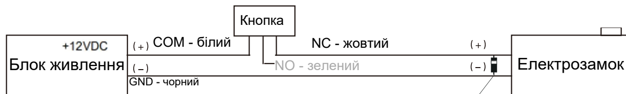
Пример подключения Fail Safe замка
