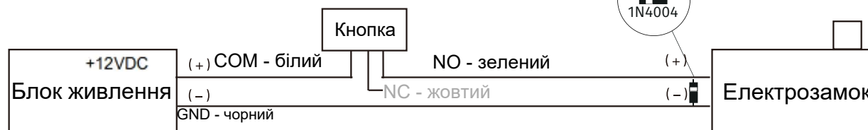
Пример подключения Fail Secure замка
