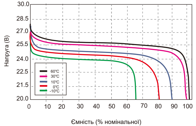
Крива розряду при різних температурах при 0.5C
