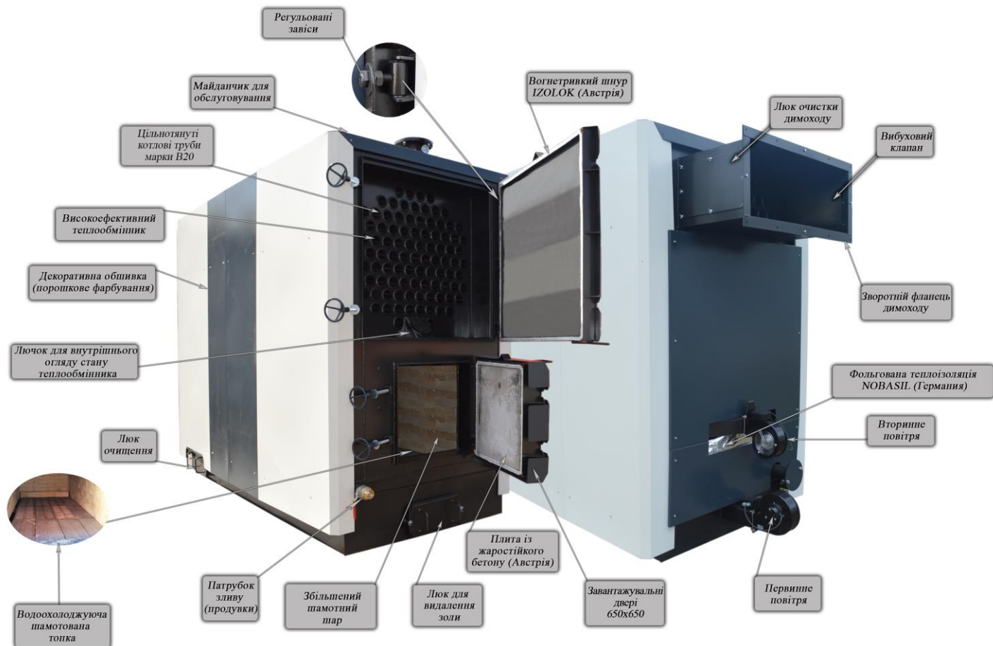
Рис.1 Основні елементи котла ARS 100-1250 SP-A (ARS 100-2000 SP-LM)
