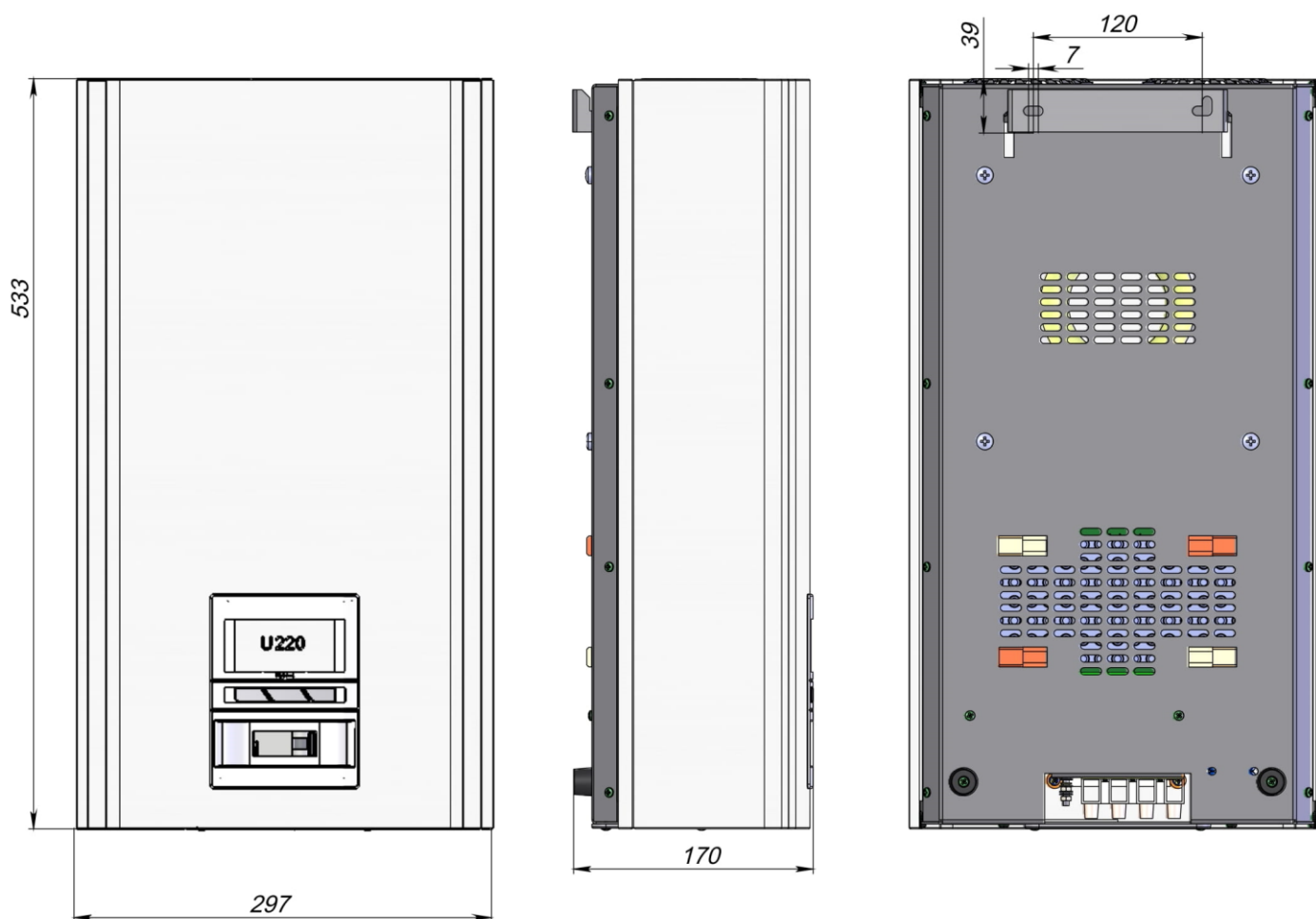
Рисунок 5. Установчі та габаритні розміри стабілізатора
