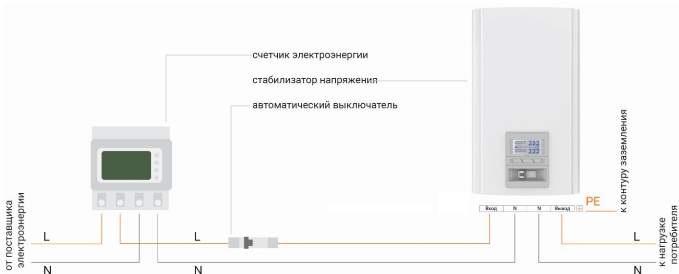
Рисунок 6. Схема подключения КилоГерц к однофазной сети
