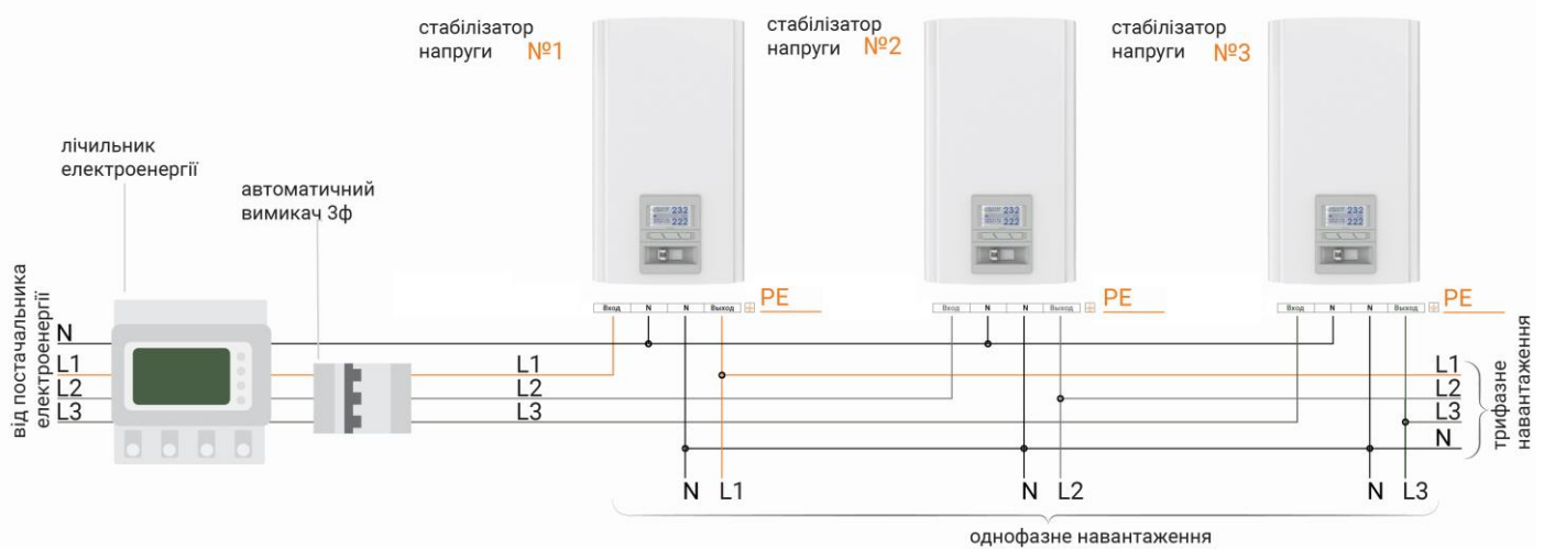
Рисунок 7. Схема підключення стабілізатора до трифазної мережі
