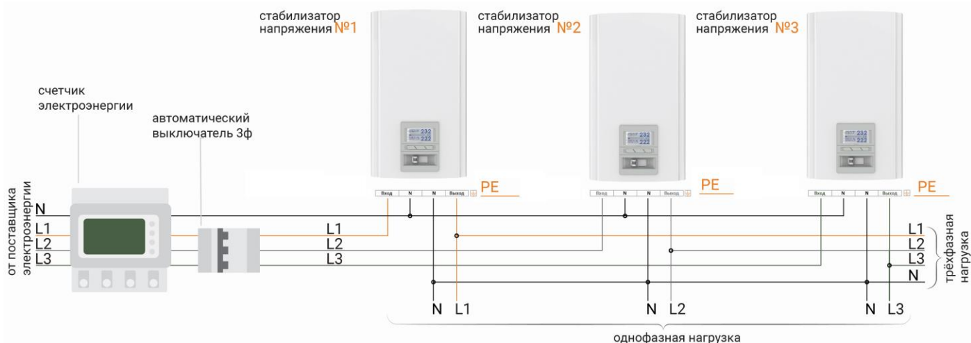
Рисунок 7. Схема подключения КилоГерц к трёхфазной сети
