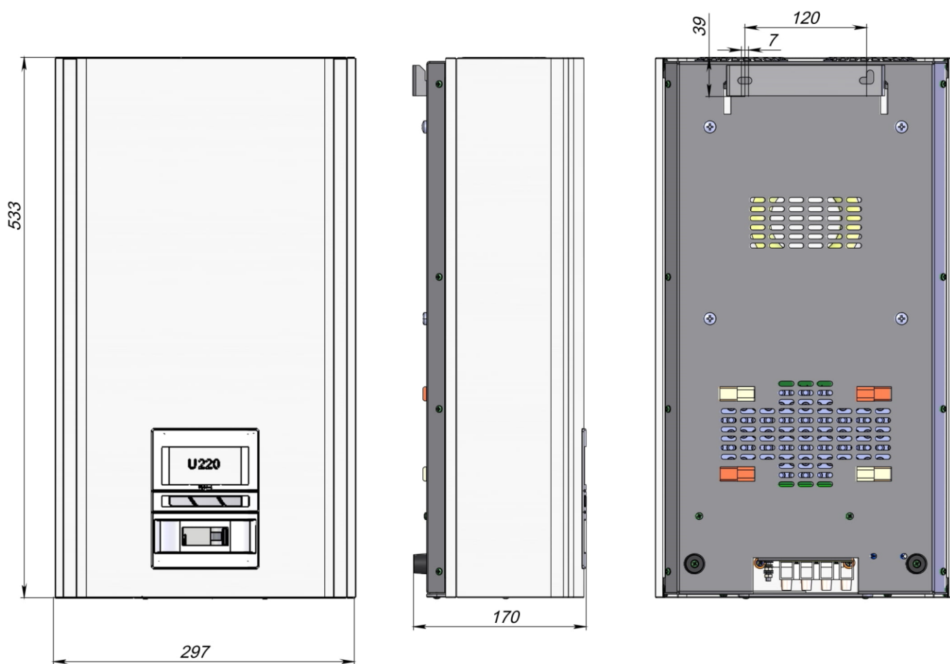
Рисунок 4. Крепление стабилизатора на установочную планку
