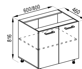
H 60/80 D 60/80
