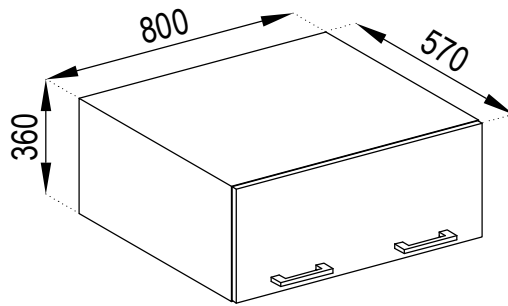
A 80 (570) HC 80 (570)
