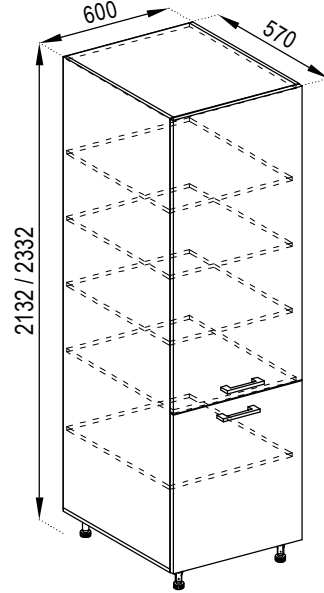
П 60 (720/920) С 60 (720/920)
