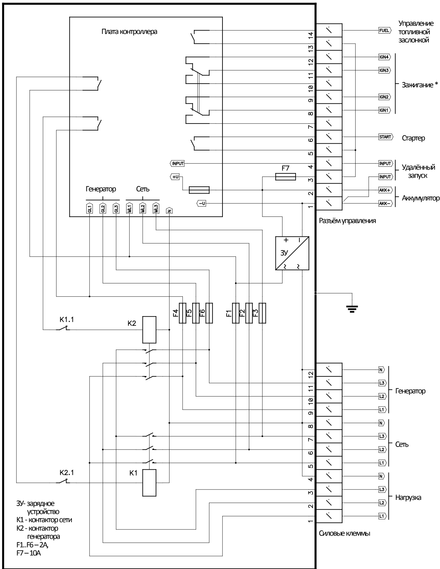
Рис 6.3 Пример схемы подключения контроллера AVR33CE.
