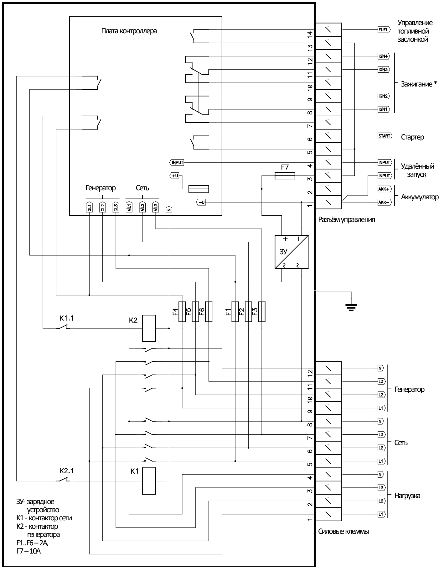
Рис 6.2. Пример схемы подключения контроллера AVR33ME.
