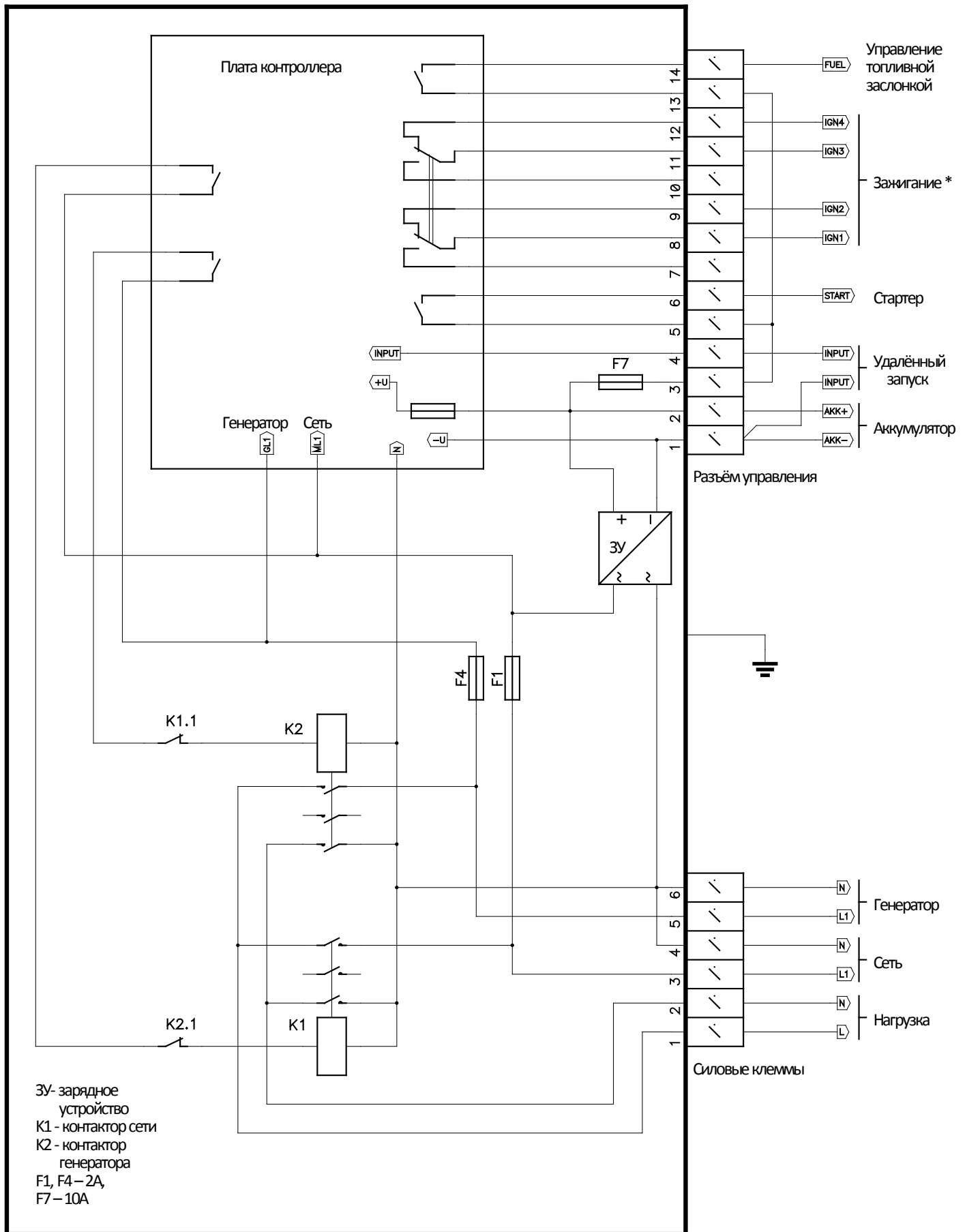
Рис 6.2. Пример схемы подключения контроллера ABP11ME / ABP11CE.
