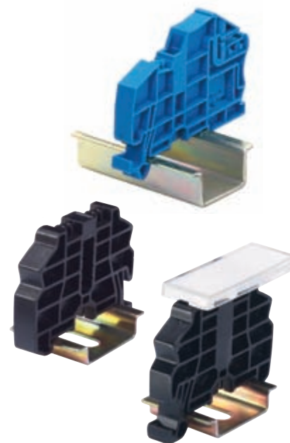
Концевая скоба для TS 35 с безвинтовым креплением
