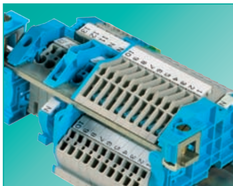
Сборная шина
