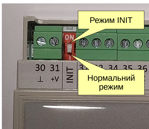
Рисунок 15 – Перемикач INIT
