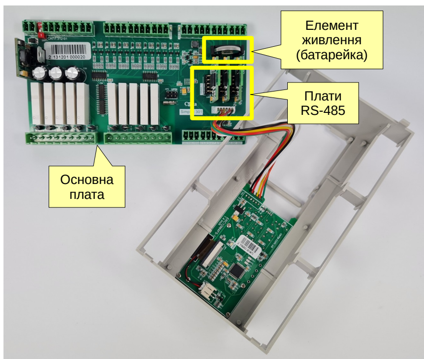
Рисунок 8 -Розібраний контролер
