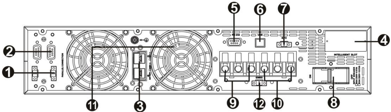
Рисунок 1. Задняя панель ИБП CORE 6-10K
