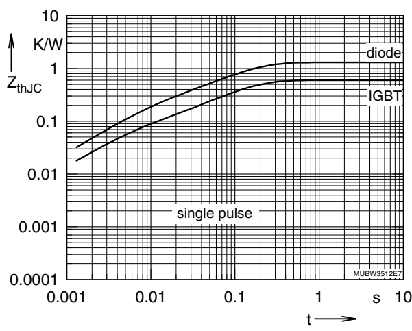
Fig. 6 Typ. transient thermal impedance
