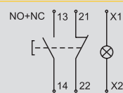
Электрическая схема
