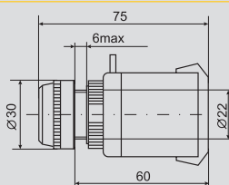
Габаритные размеры
