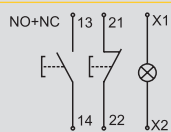
Электрическая схема
