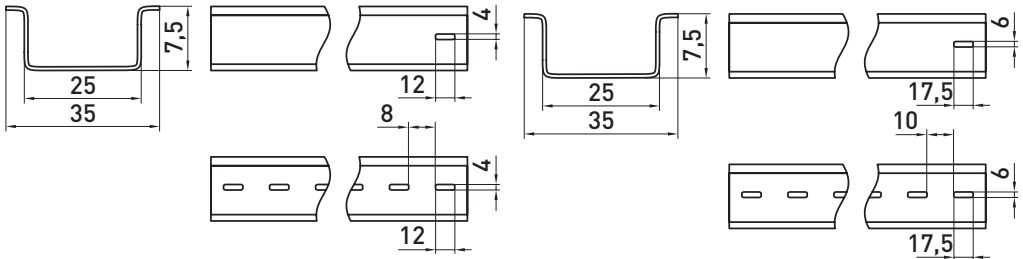
Рис. 1 e.din.stand.rail.101 e.din.stand.rail.102
