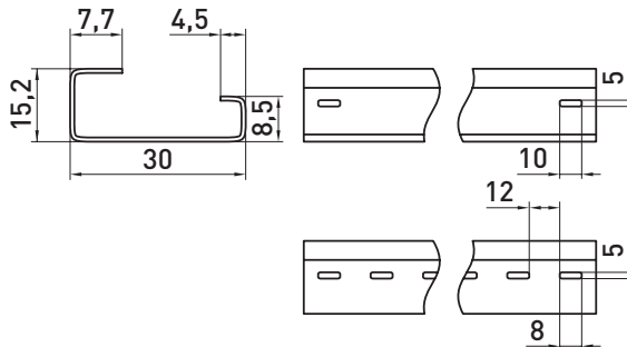
Рис. 3 e.din.stand.rail.301 e.din.stand.rail.302
