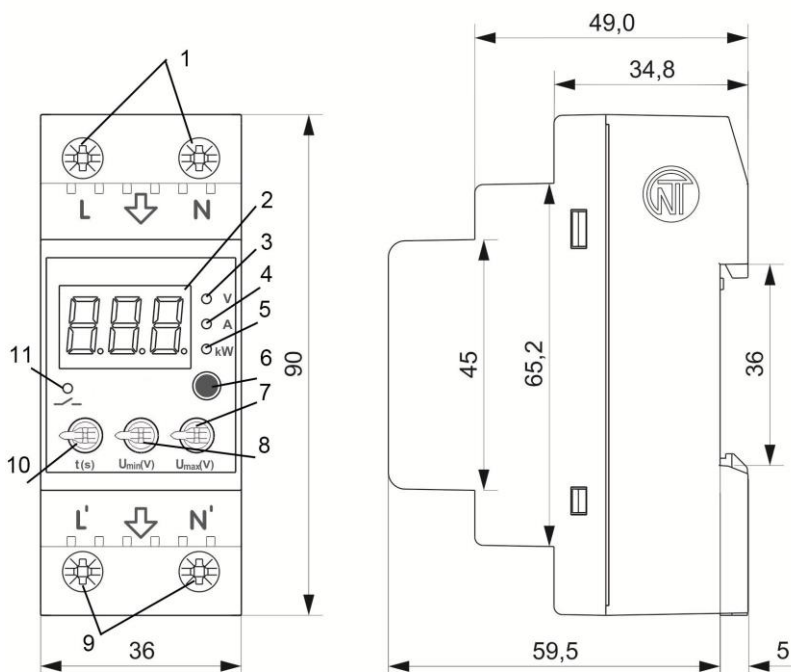
Рисунок 1 – Органы управления и габаритные размеры РН-263t
