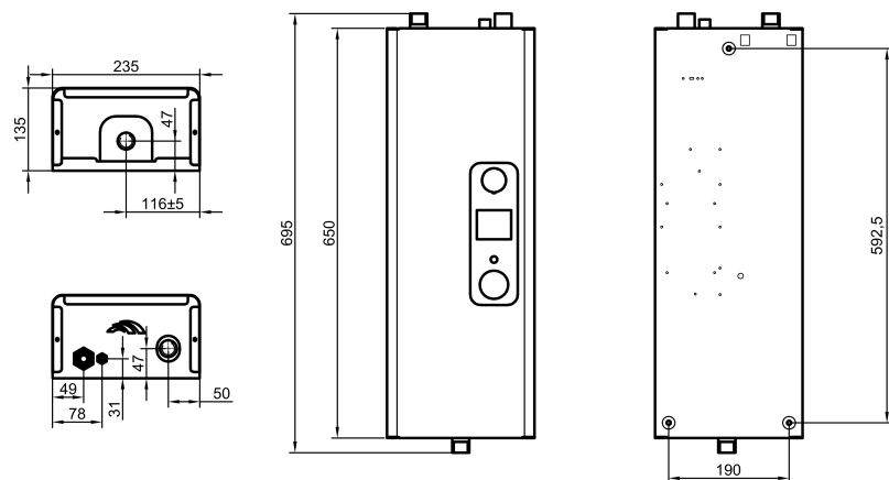
Рисунок 2 - Апарат КЕО-4,5-15 кВт (230В; 400В) - Б м
