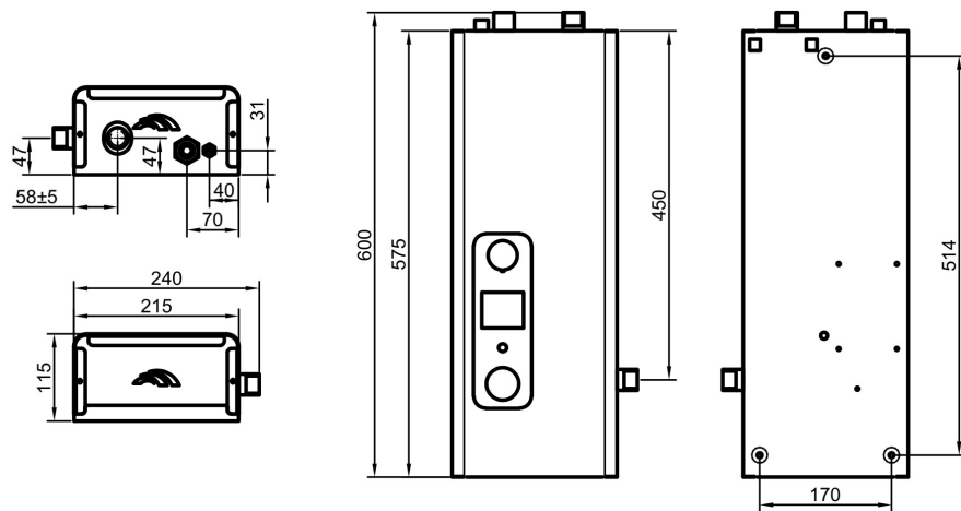
Рисунок 2 – Апарат електричний водогрійний «Дніпро»
