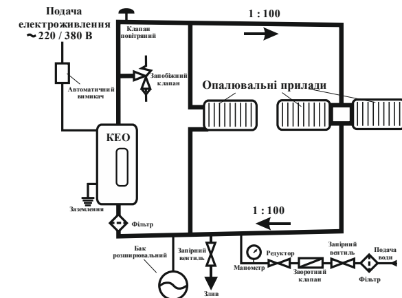
Рисунок 1 -Рекомендована принципова схема системи опалення
