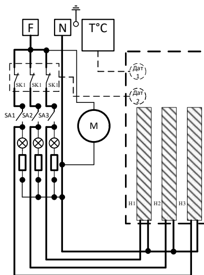
Рисунок 3 - Схеми електричні принципові КЕО-МБ 4,5-12/(220)380
