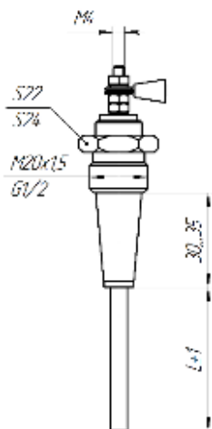
Рисунок 1 - Габаритні розміри ДУ
