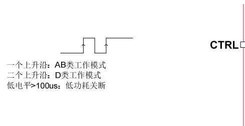
图4 NS4160 工作模式设置
