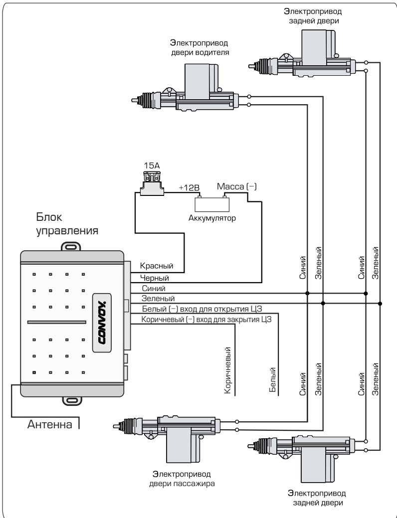
Схема подключения к двухпроводным приводам
