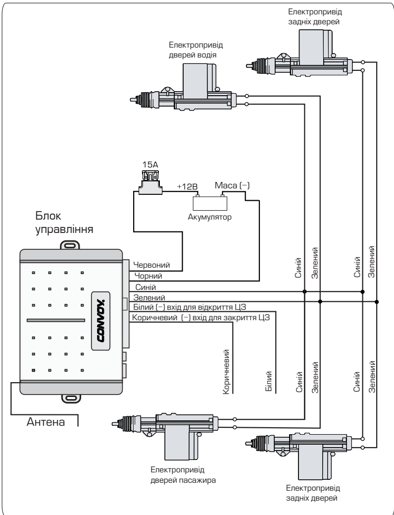
Схема підключення до двопроводних приводів
