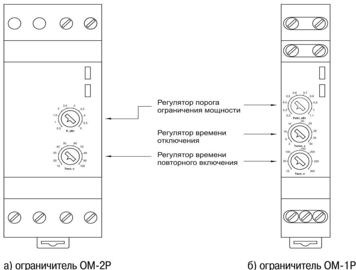
Рисунок 2 – Регуляторы ограничителей
