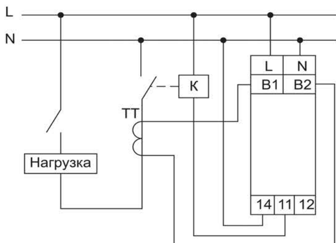
Рисунок 3 – Схема подключения ограничителя ОМ-1Р
