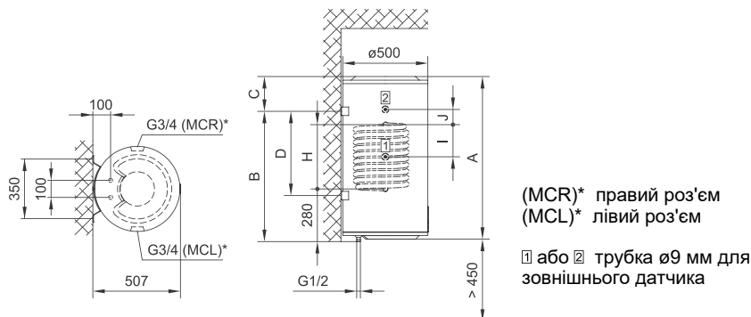
Мал. 1: Монтаж на стіну у вертикальному положенні
