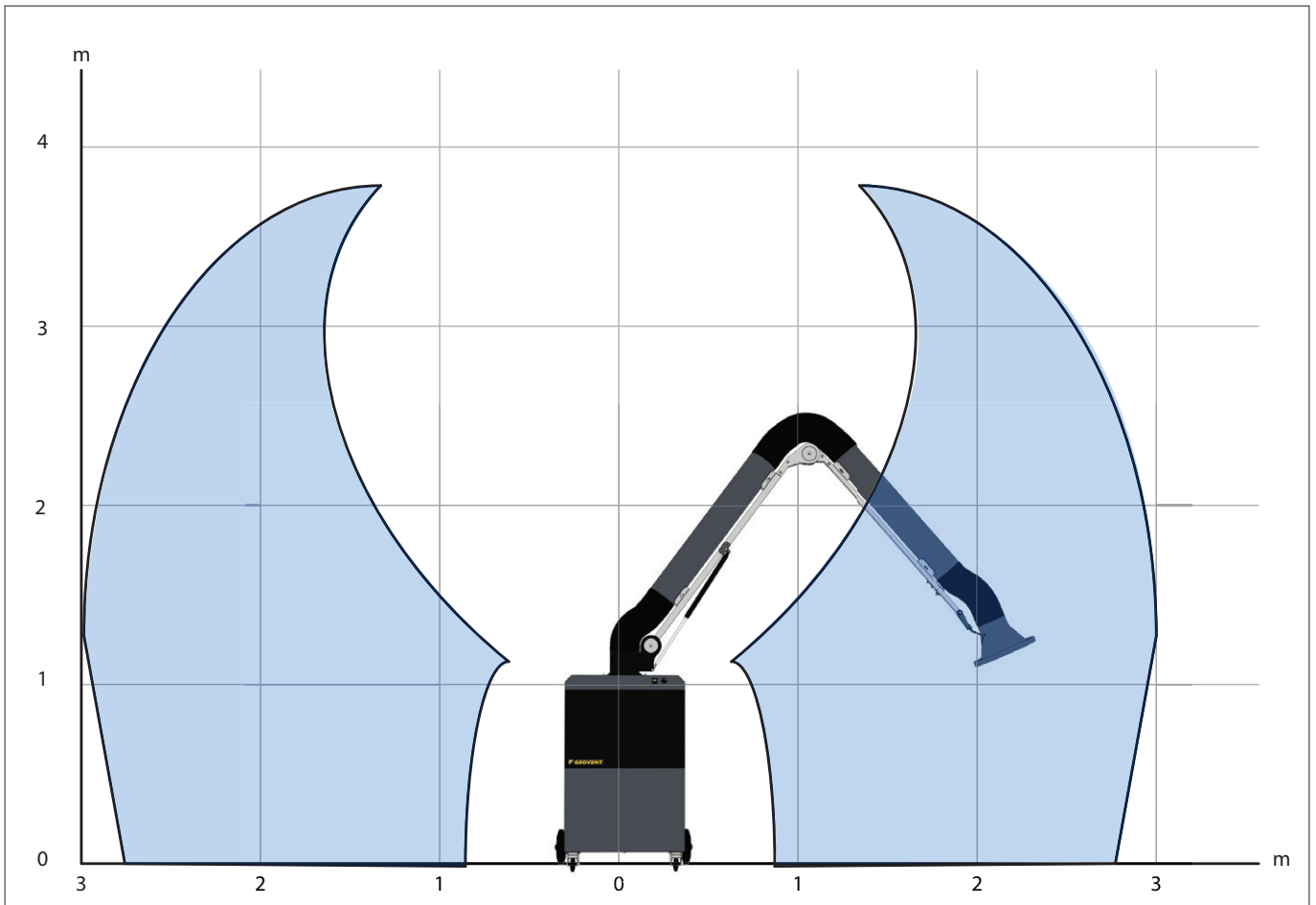
Робоча зона для GeoGo з маніпулятором ASA4o with ASA4 arm
