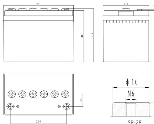
Габаритні розміри, мм
