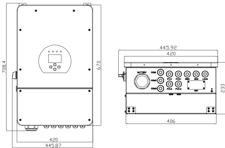
Розмір інвертора
