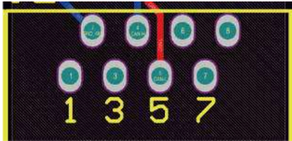
CAN Порт
