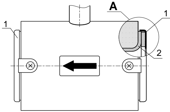
ПТР с защитными кольцами
