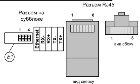
Рис.А.8. Обозначения коммутационных элементов на субблоке вычислителя.
