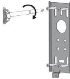
Мал. 5 Задній кронштейн
