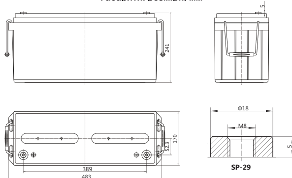
Габаритні розміри, мм
