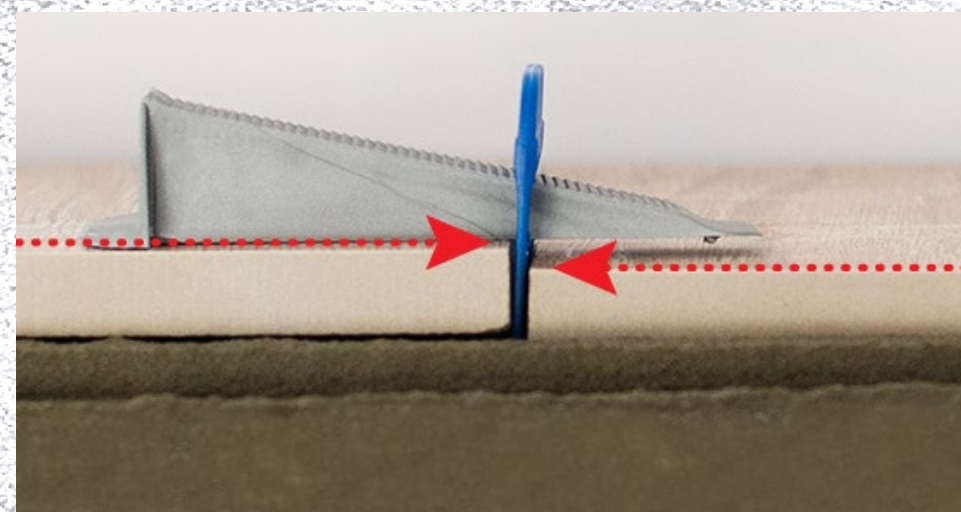
В зажим вставляється універсальний клин
