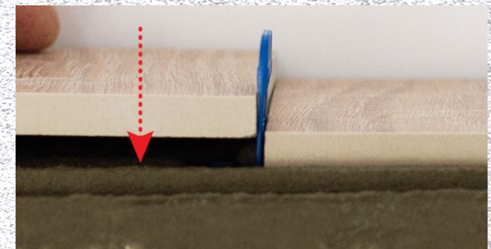
Зверху, поверх лапок зажиму, встановлюється друга плитка, впритул до попередньої
