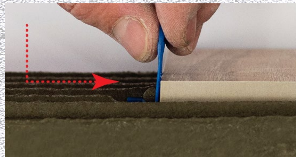
Після встановлення першої плитки під неї встановлюється зажим
