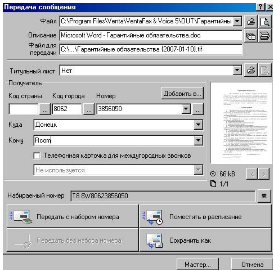
Рис. 9.6 – Окно передача факсимильного сообщения
