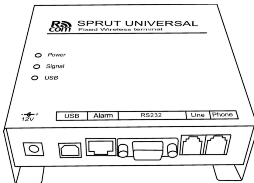
Рис. 1 Внешний вид устройства
