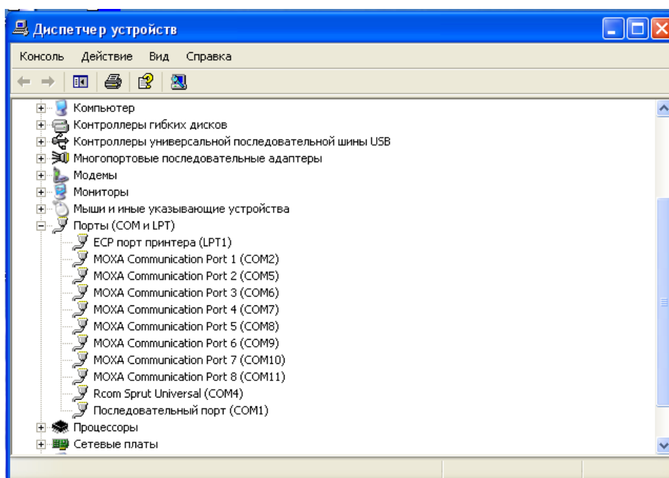
Рис. 7.6 – Диспетчер устройств
