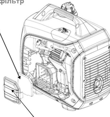
Повітряний фільтр
