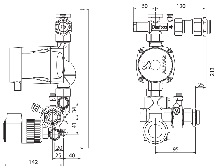
Рис. 14: FHM-C7 с термоэлектрическим приводом ABV для реализации функции погодной компенсации
