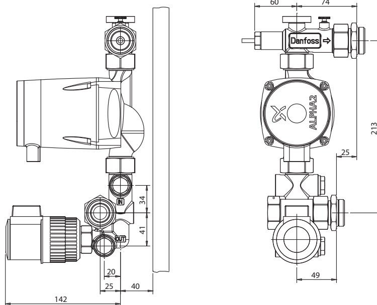
Рис. 16: FHM-C8 и FHM-C9 с термoeлектрическим приводом ABV для реализации функции погодной компенсации
