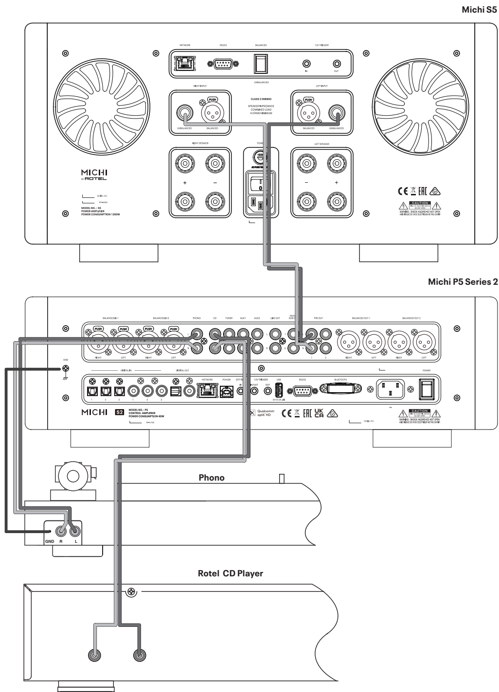
Figure 4: Analog Input and Output Connections Branchements des entrées et sorties analogiques Analoge Ein- und Ausgangsanschlüsse Entradas y Salidas Analógicas Analoge ingangen en uitgangen Collegamenti ingressi ed uscite analogici Anslutningar för analoga in- och utgångar Аналоговые входы и выходы
