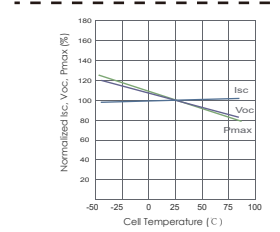
LP182*182-M-72-NH-580W
