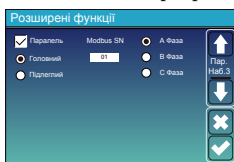
Головний інвертор
