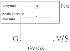
GV/GS (сигнал запуску дизельного генератора)
