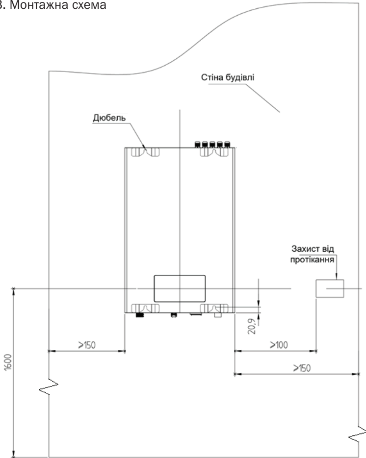
Рис. 3. Монтажна схема
