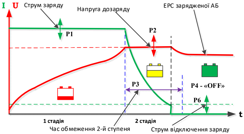
Рис.3в. Вимкнення при зниженні струму дозаряду до встановленого значення.
