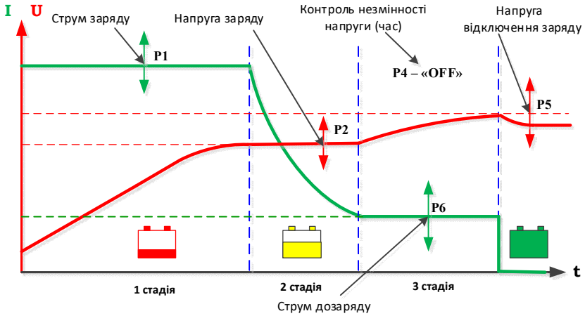
Рис.4а. Вимкнення при досягненні максимальної напруги
