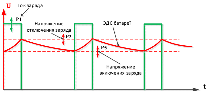
Рис.3д. Періодичний підтримуючий заряд батареї.
