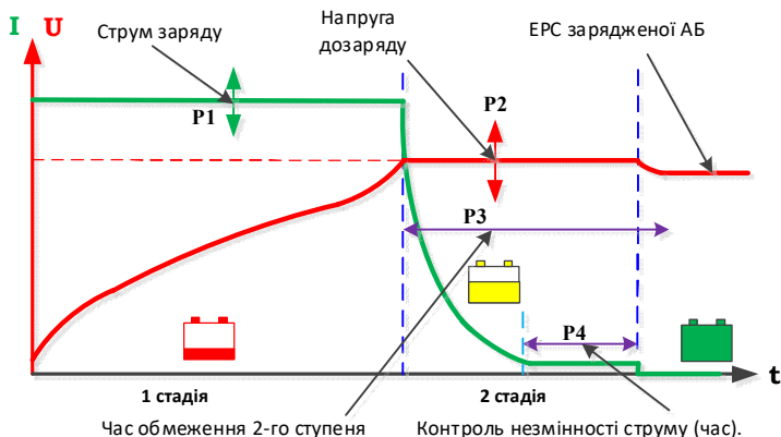
Рис.3г. Вимкнення за незмінністю струму дозаряду протягом встановленого часу.
