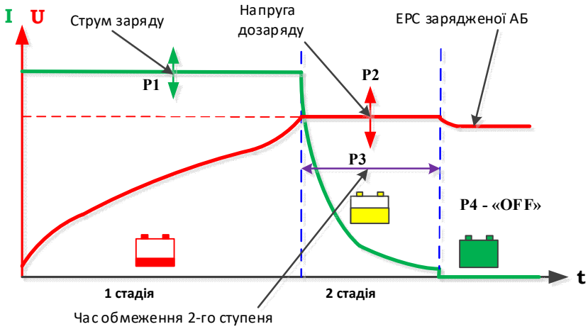
Рис.3б. Вимкнення після закінчення часу дозарядання.
