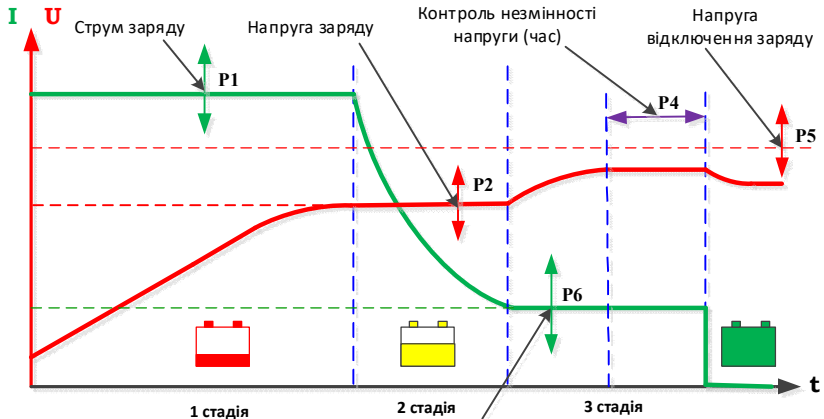
Рис.4б. Вимкнення за незмінністю напруги АБ у процесі дозарядження.
