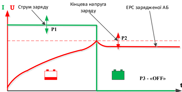
Рис.3а. Вимкнення після досягнення кінцевої напруги
