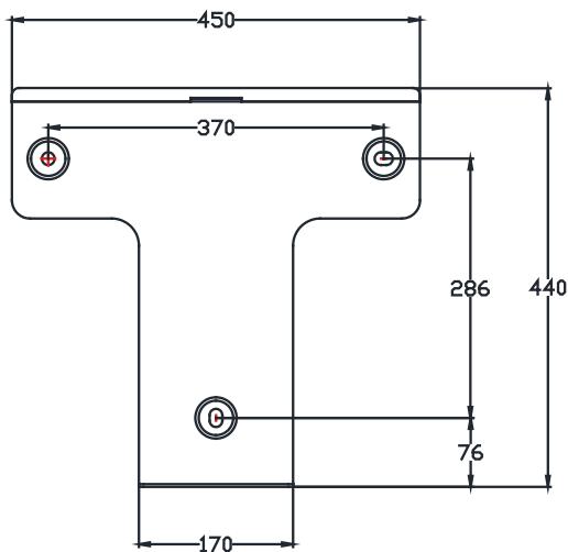
Рис. 4.4 Розміри монтажного кронштейна
