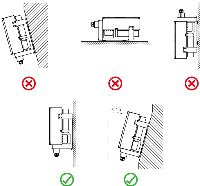
Рис. 4.2 Кут встановлення
