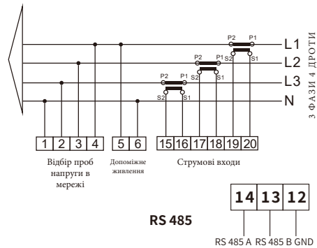
Рис. 7.7 Лічильник Eastron
