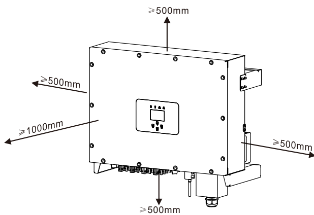
Рис. 4.3 Монтажний проміжок
