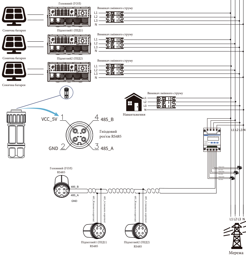
Рис. 7.33 Схема підключення CHNT (таблиця пропускнуної здатності)
