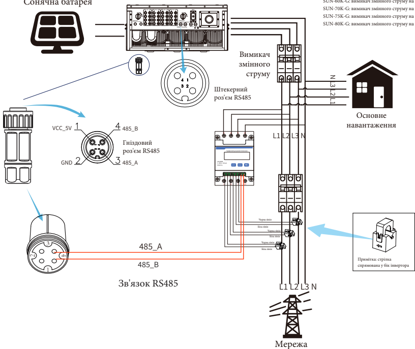
Рис. 7.14 Схема підключення лічильника CHNT
