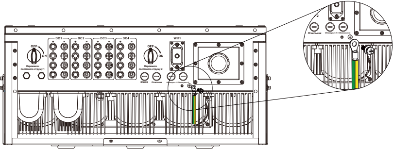
Рис. 5.12 Встановлення оболонки дроту заземлення
