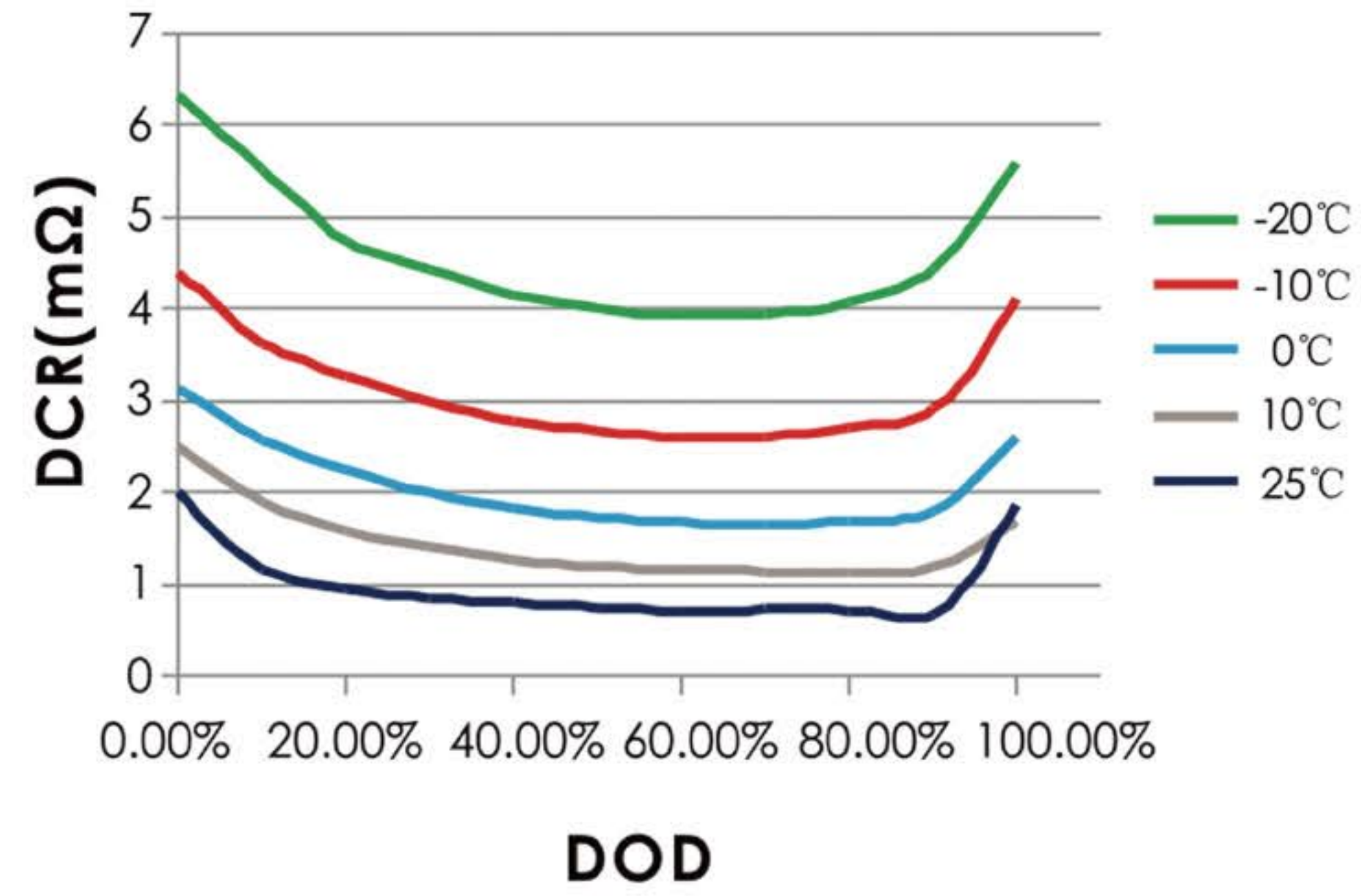
DCR Test
