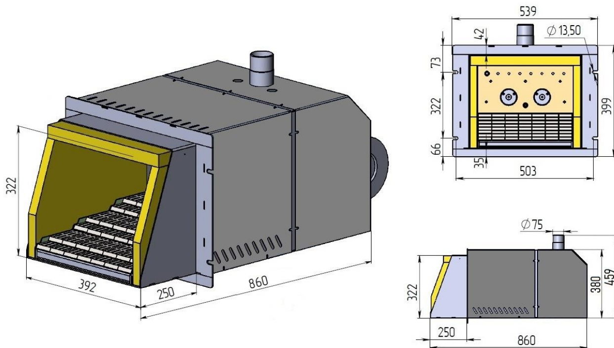
Мал. 1 - Габаритні розміри пальника «SPARK» 200 кВт
