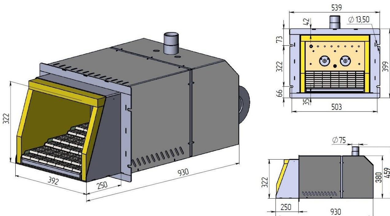
Мал. 1 - Габаритні розміри пальника «SPARK» 200 кВт
