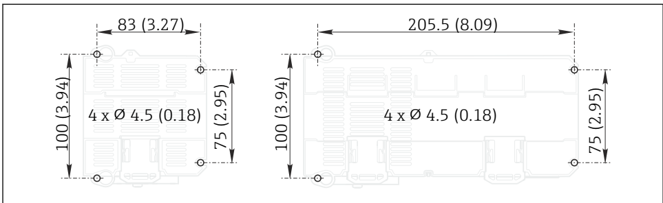
2 Схема отверстий для настенного монтажа в мм (дюймах)
