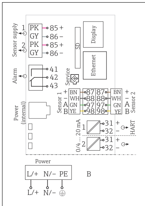
8 Полная электрическая схема на примере модуля BASE2-E и внешнего блока питания (B)
