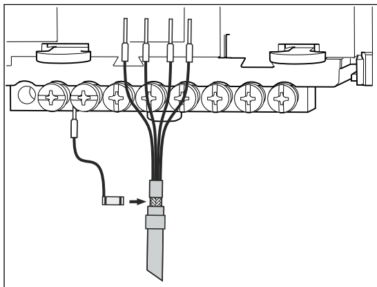
9 Подключение функционального заземления
