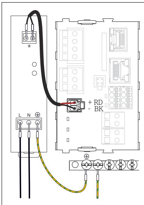
7 Подключение электропитания на примере модуля BASE2-E
