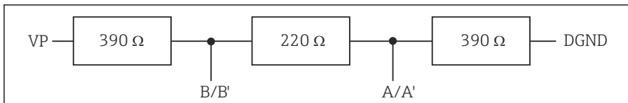
31 Структура внутреннего терминирования
