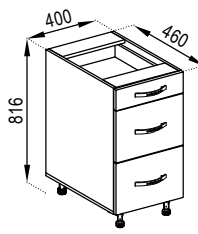
H 40 Ш D 40 Dr
