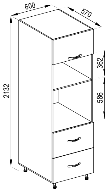
П 60 ДШ (920) під духовку і мікрохвильову С 60 DDr (920) for oven & microwave
