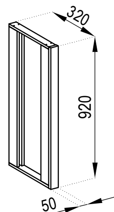
В вставка (920) U insert (920)
