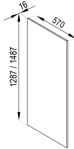
П Панель внутрішня (720/920) C Panel internal (720/920)
